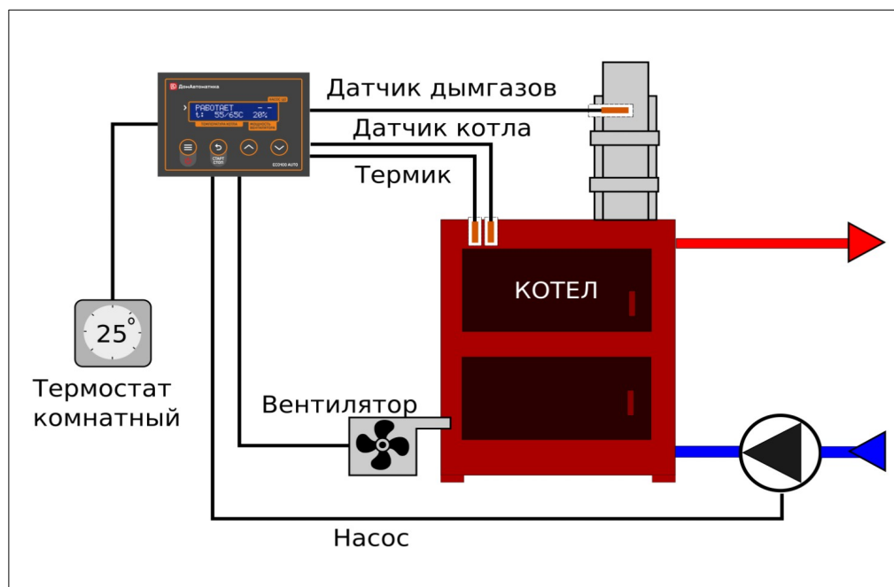
Рисунок 2 - Схема подключения контроллера ЕСО100 к котлу.
